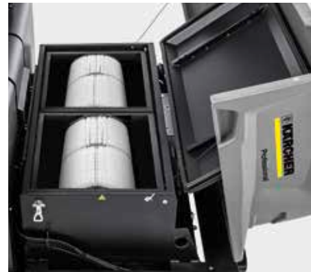
Rundfilter
